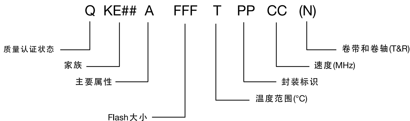
图2. 部件编号图
